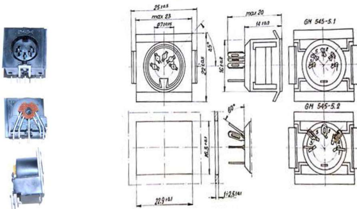
Wymiary otworu płyty montażowej
